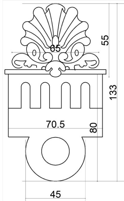
B - Remate motivo hojas sobre tablero replanado con moldura. Cantidad a reproducir: 6
