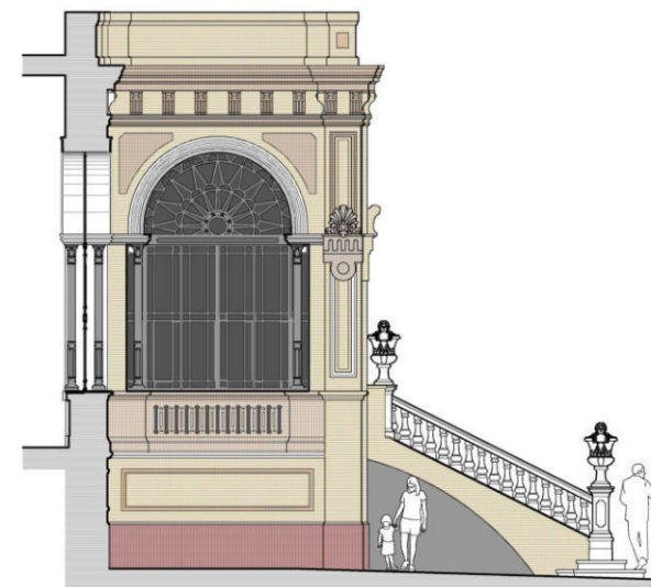
Fachada lateral Oeste
