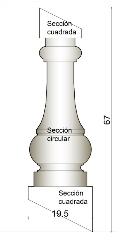
C - Balaustre original en mármol a reproducir en material de albañilería con terminación lustrada Cantidad a reproducir: 32
