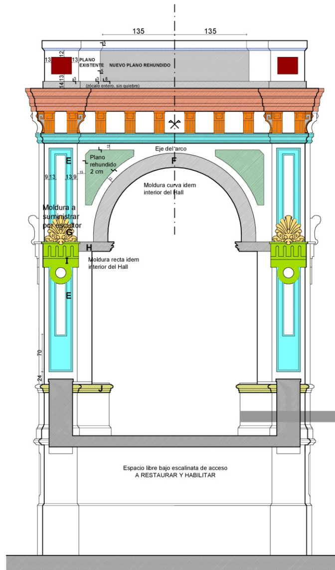
C Fachada principal Sur ACCESO
