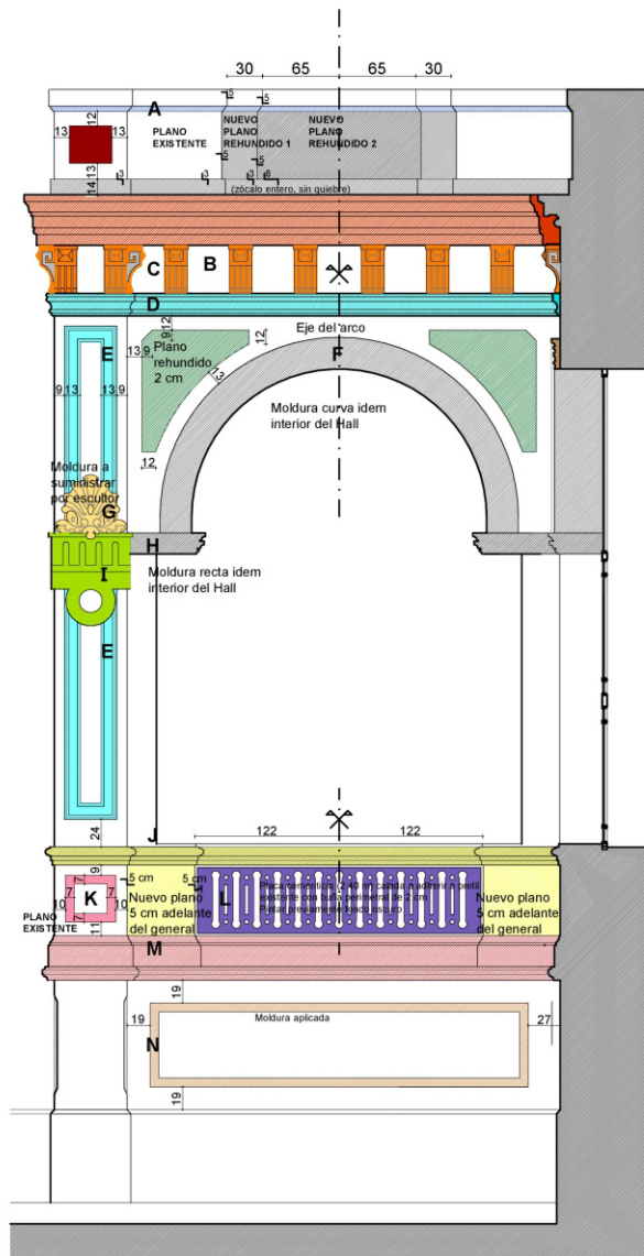
A Fachada principal Sur PLANO POSTERIOR izquierdo
