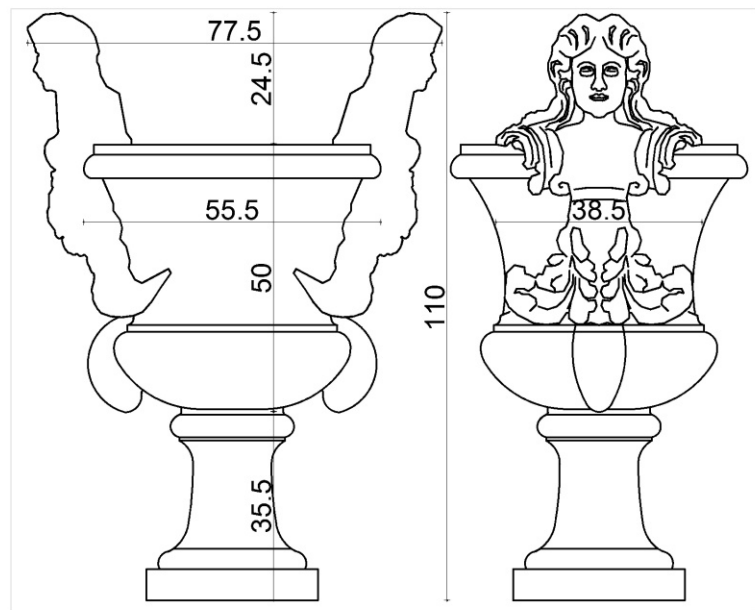
D - Macetero ánfora. Cantidad a reproducir: 4 (se utilizala existente para la toma del molde)
