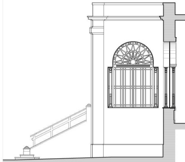
Fachada lateral Este
