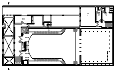
PLANTA NIVEL 1
